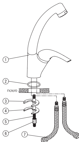
מפרט חלקים:
