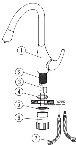
מפרט חלקים:
